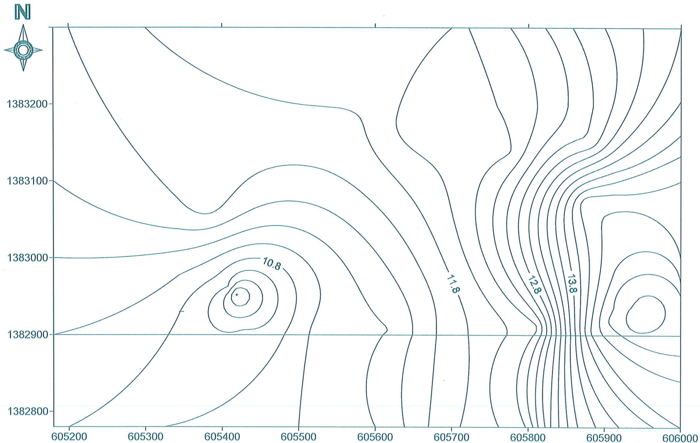
แสดงเส้นชั้นความสูง (ม.รทก.) 1:3,000
